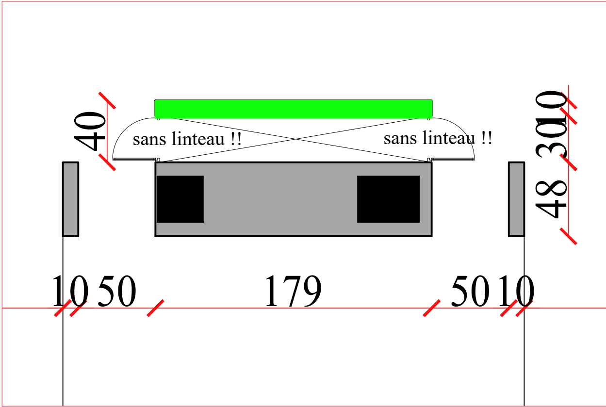
Plan de construction maçonnerie Stockage toiles
