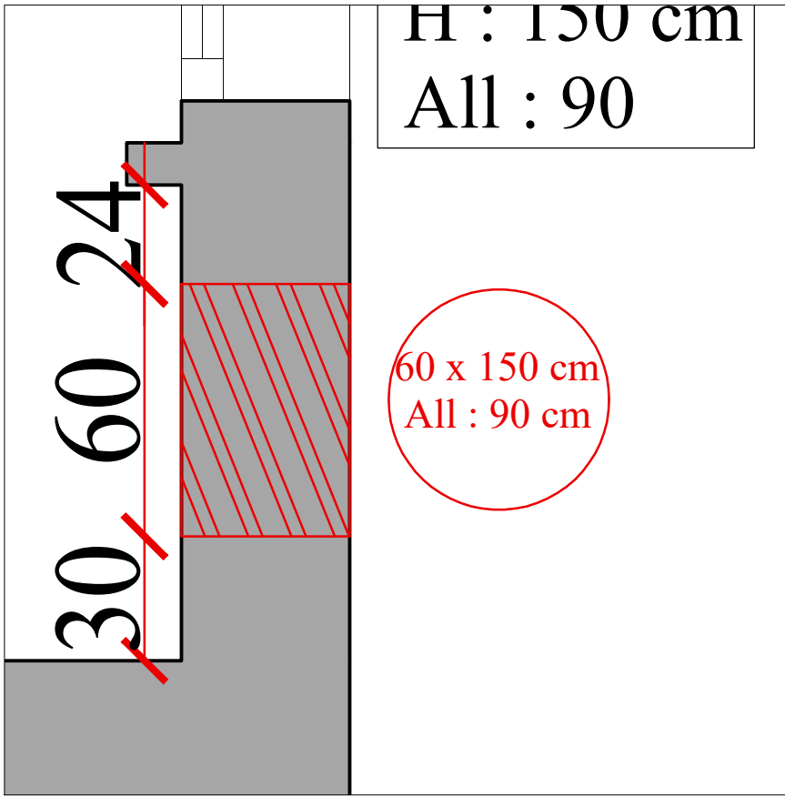
Plan de démolition de la fenêtre SDE invités
