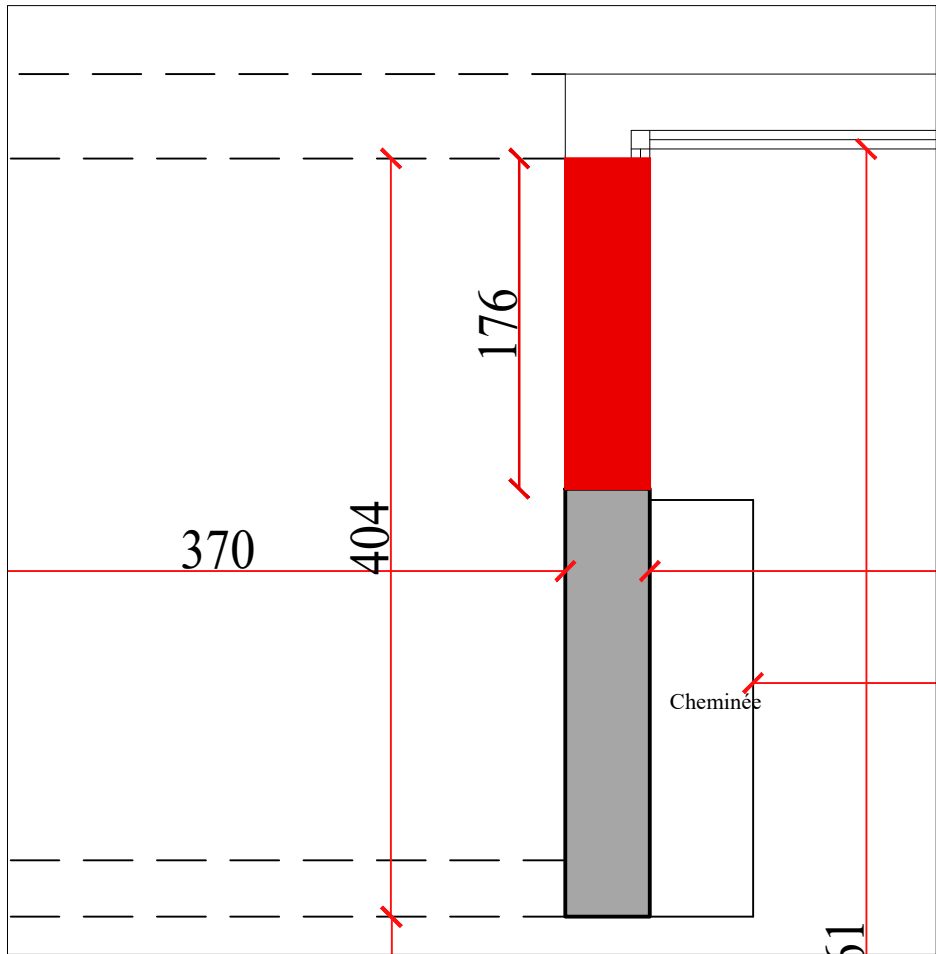
Plan de démolition mur salon
