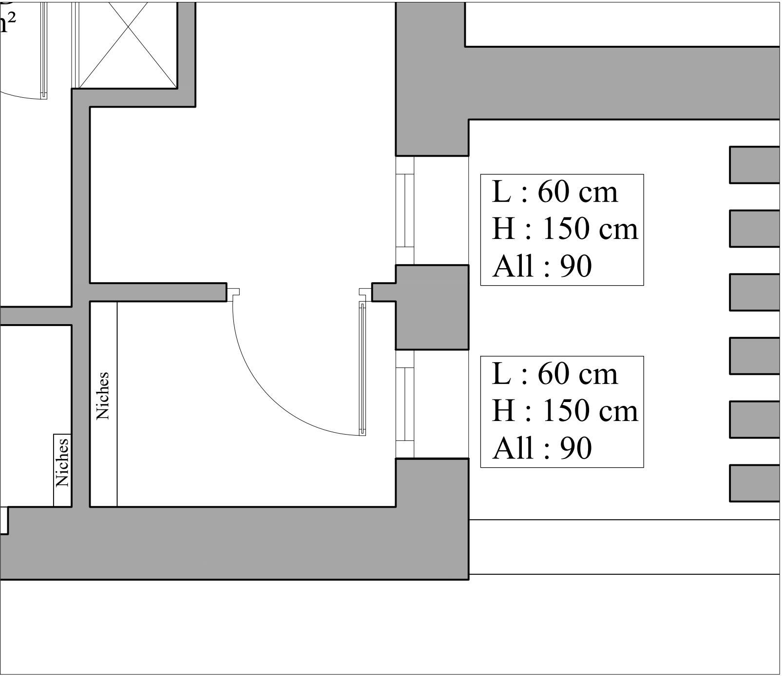
Repérage sur plan (SDE invités)
