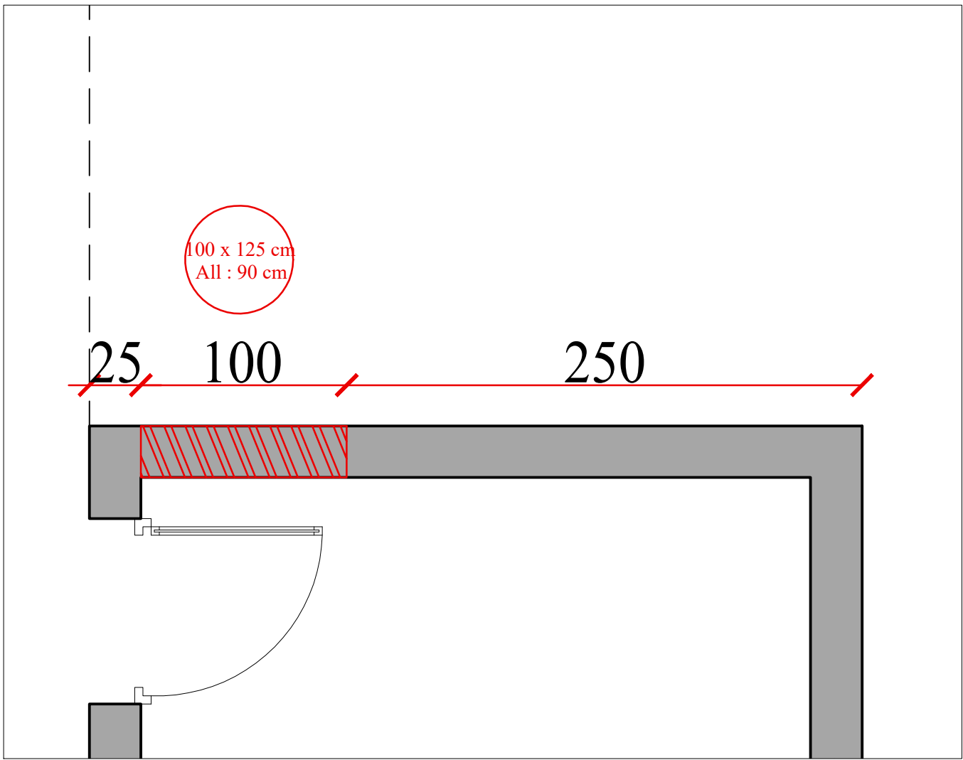
Plan de démolition des fenêtres Local Technique
