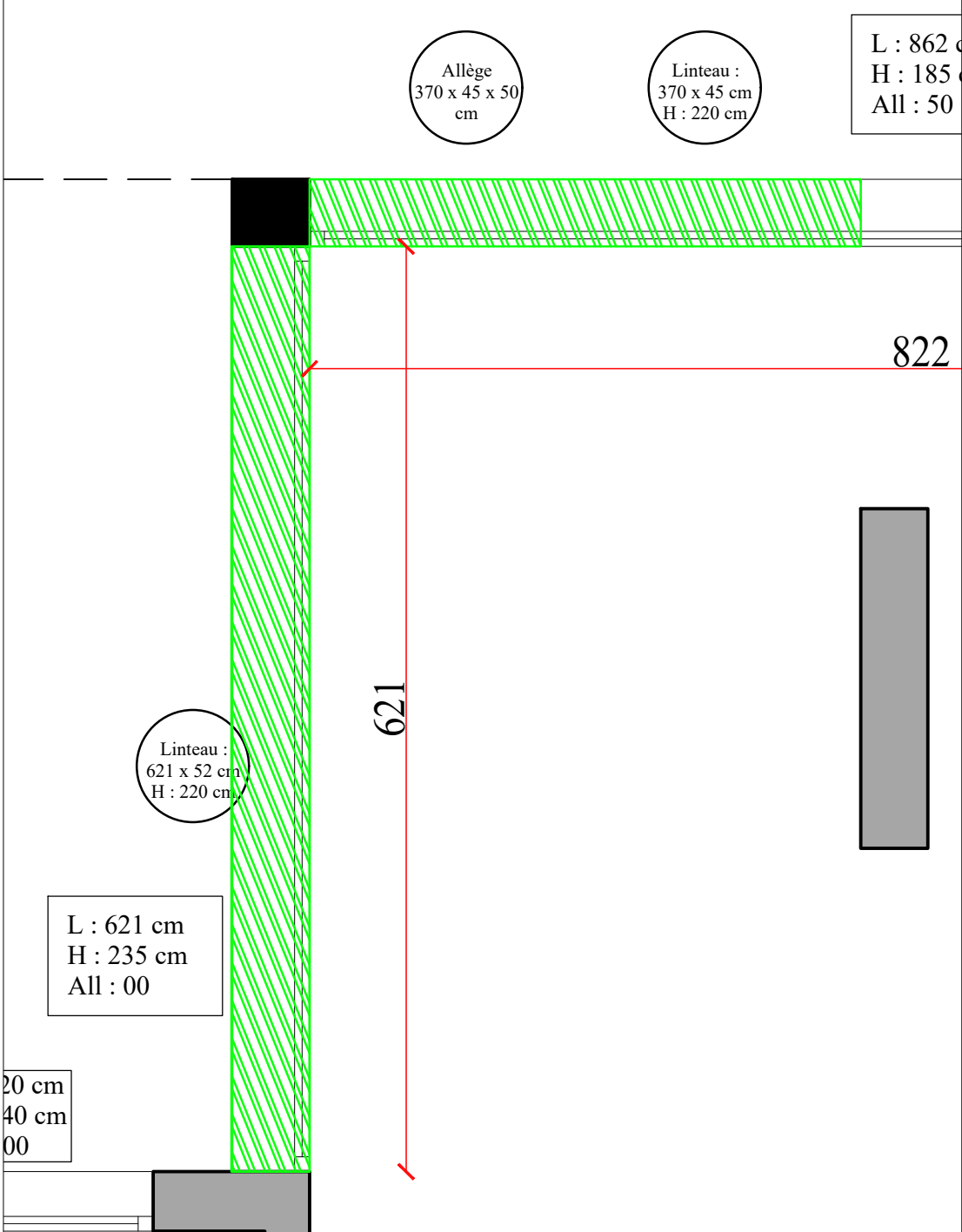
Plan de construction maçonnerie Salon
