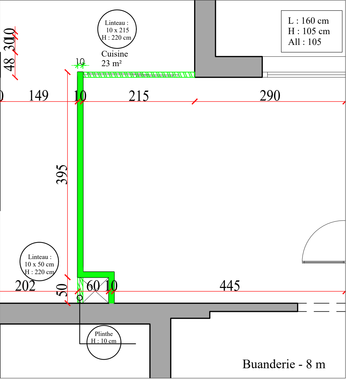
Plan de construction maçonnerie Cuisine
