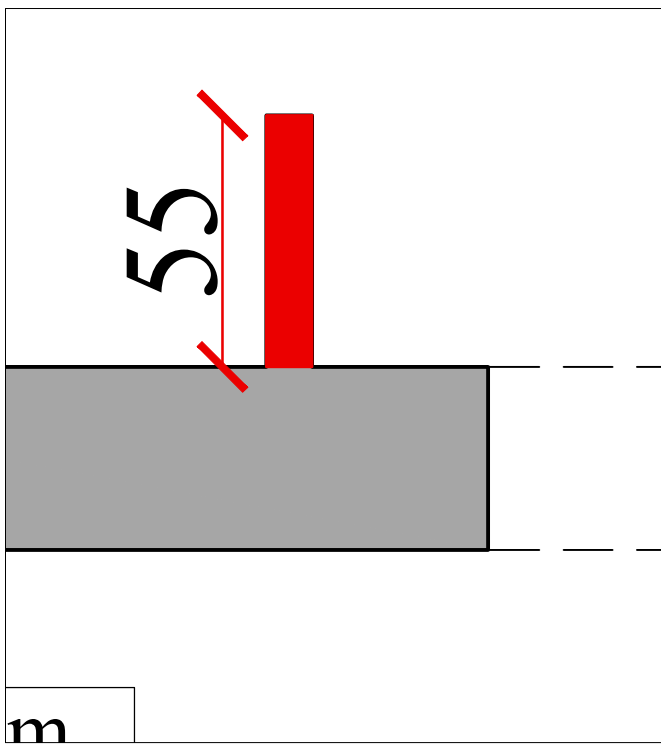
Plan de démolition mur coté entrée
