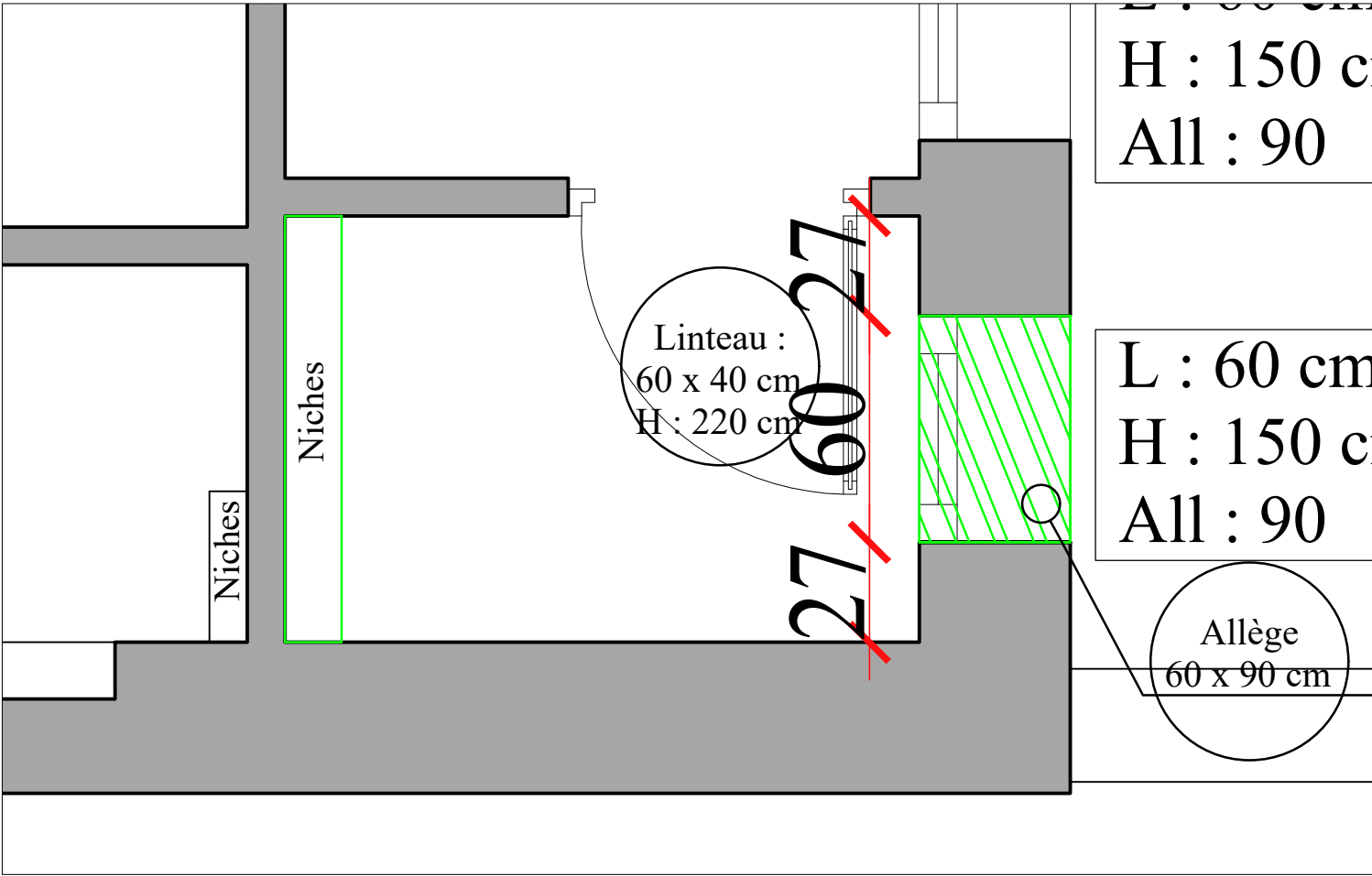
Plan de construction maçonnerie SDE invités (Voir détails Coupes)
