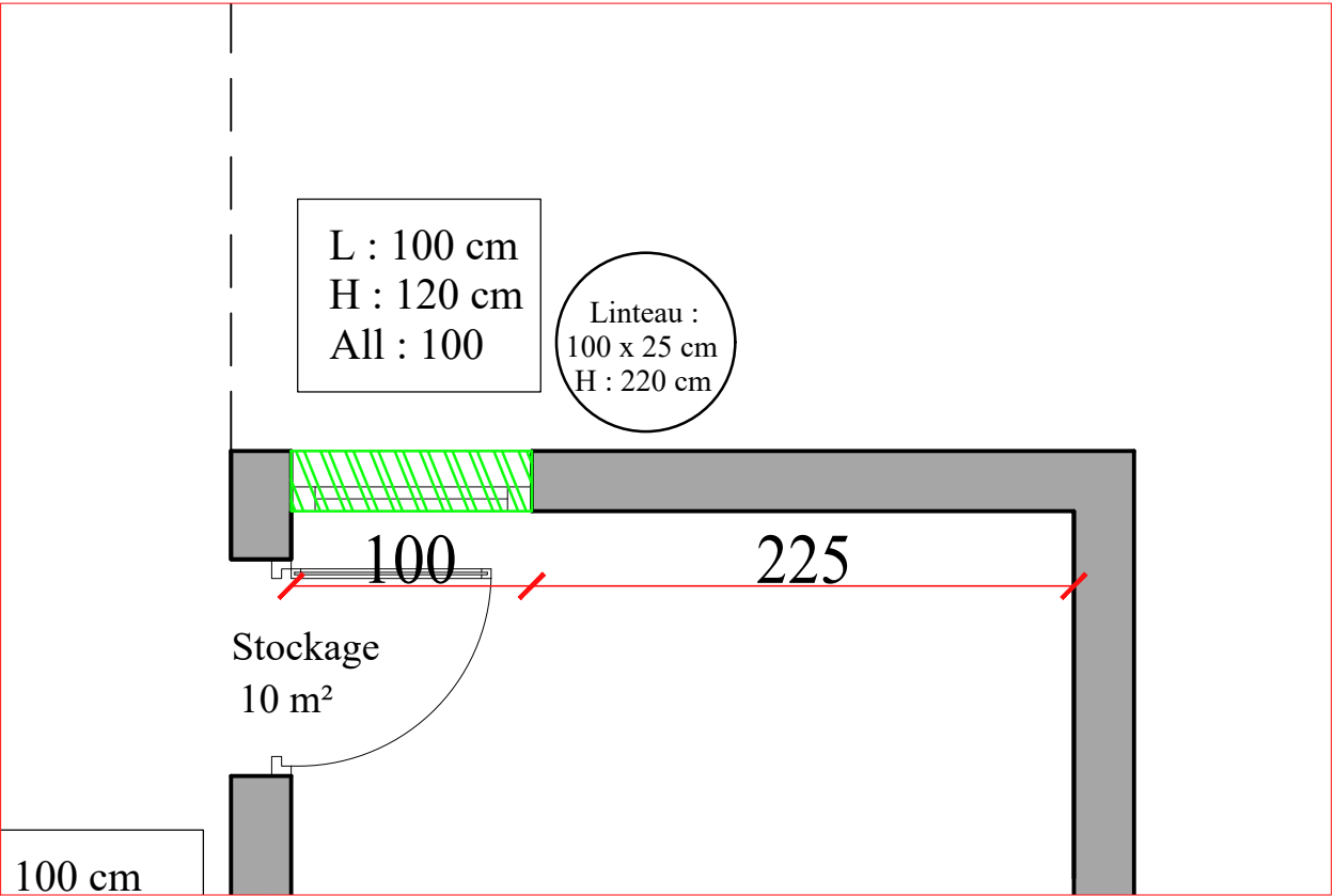
Plan de construction maçonnerie Stockage
