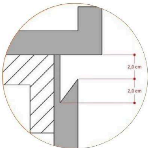
Système coupe 45°
