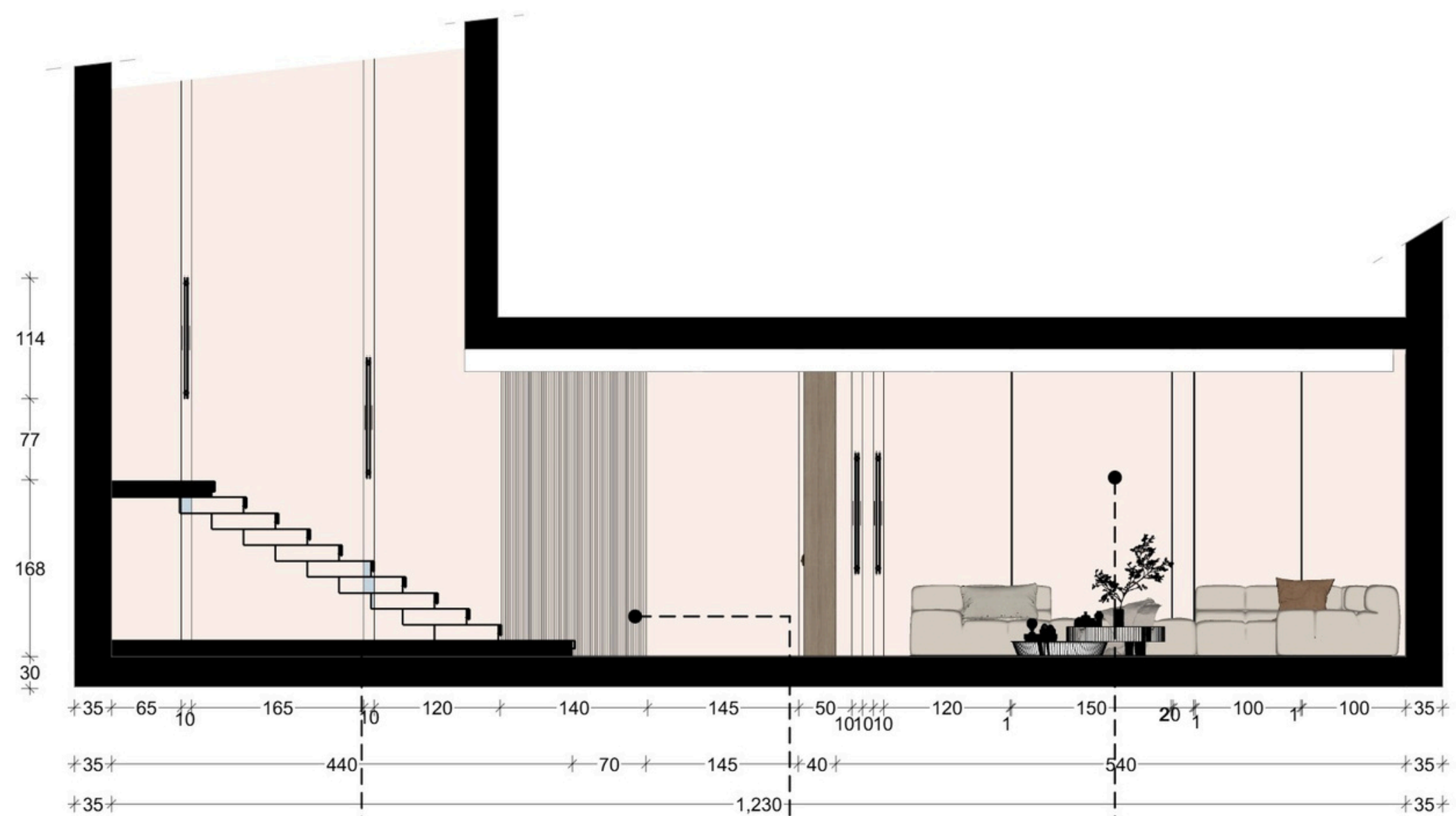
Coupe B-B
