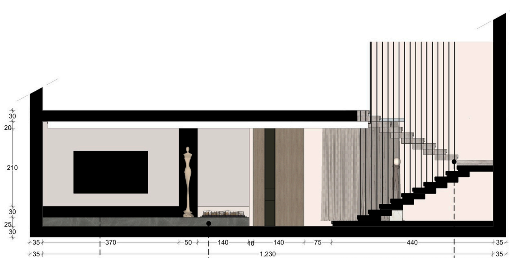
Coupe A-A
