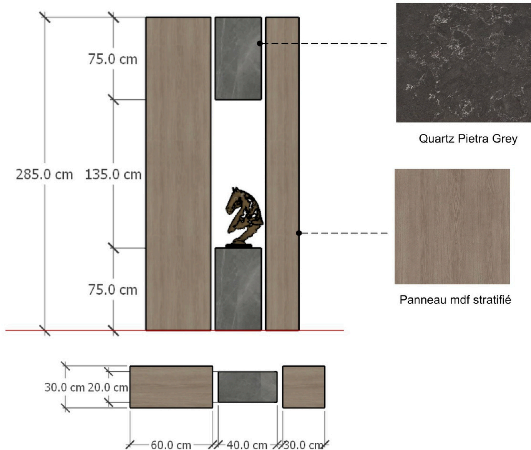
Détail séparation
